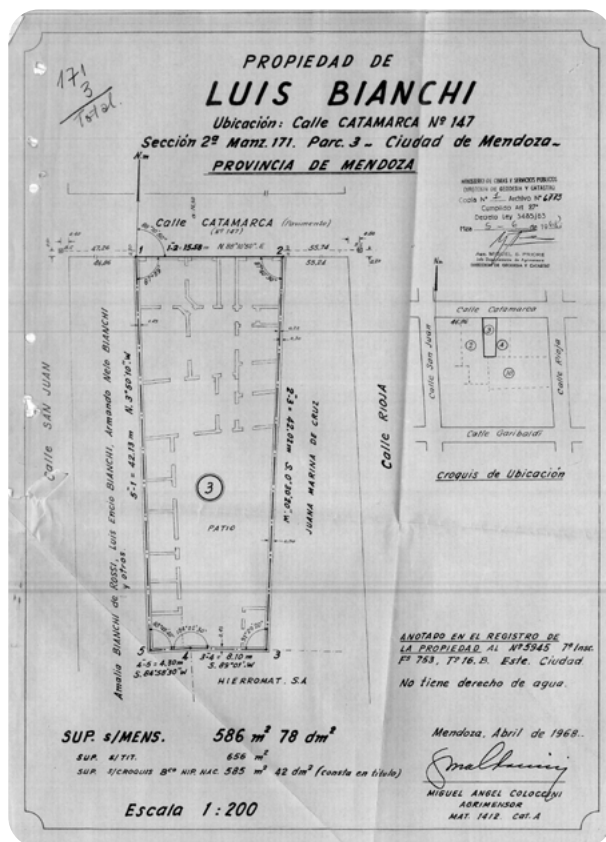
Casa Bianchi. Plano de mensura. Fuente: Dirección de Catastro, Municipalidad de Capital.
